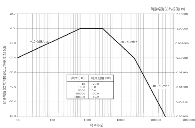
GJB 181B-2012 图13 28V直流电压最大畸变频谱
