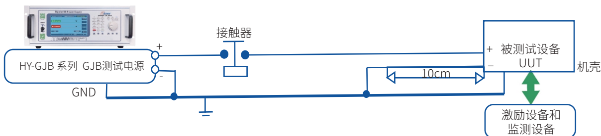
图LDC101-1 负载特性试验系统典型配置
