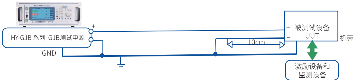
图LDC302-1 非正常电压瞬变试验系统典型配置
