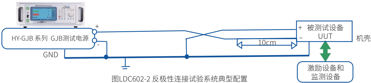
图LDC602-2 反极性连接试验系统典型配置
