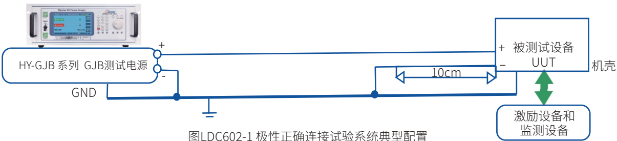
图LDC602-1 极性正确连接试验系统典型配置
