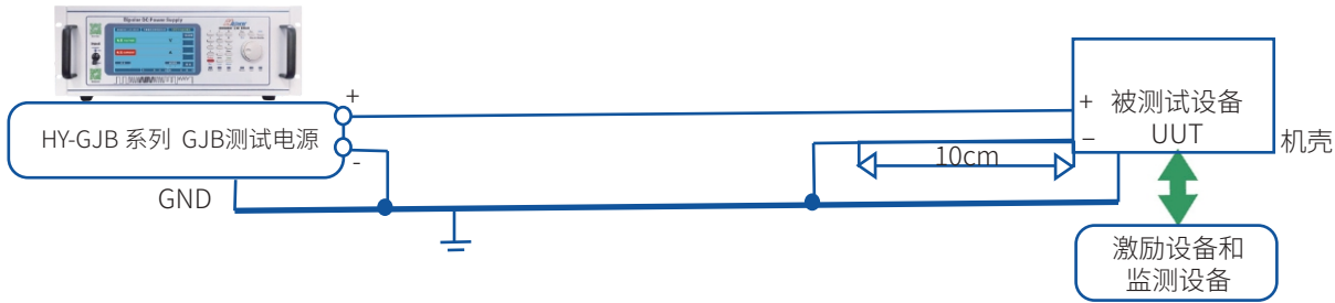
图LDC401-1 应急稳态电压试验系统典型配置
