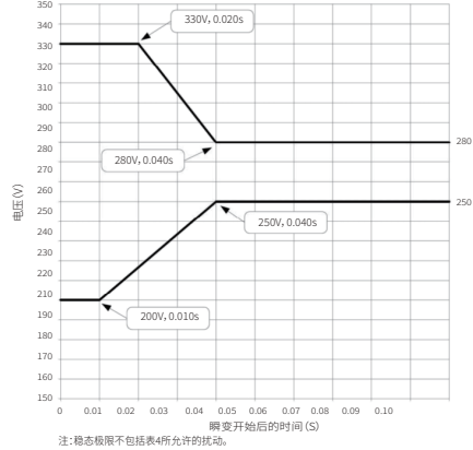
GJB 181B-2012 图15 270V直流正常瞬变电压包络线
