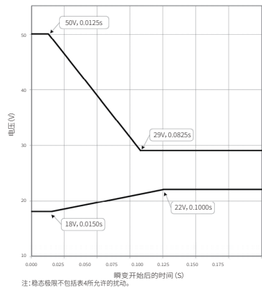
GJB 181B-2012 图12 28V直流正常瞬变电压包络线
