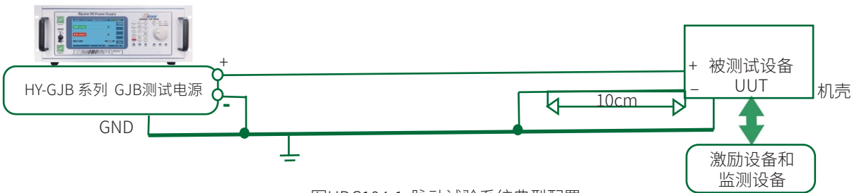
图HDC104-1 脉动试验系统典型配置
