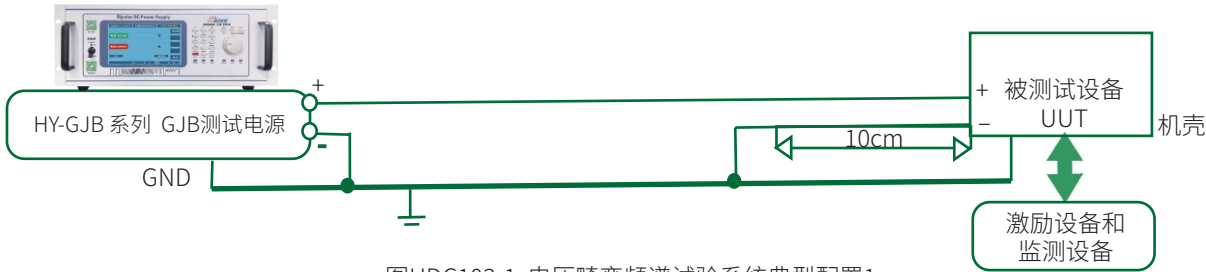
图HDC103-1 电压畸变频谱试验系统典型配置1
