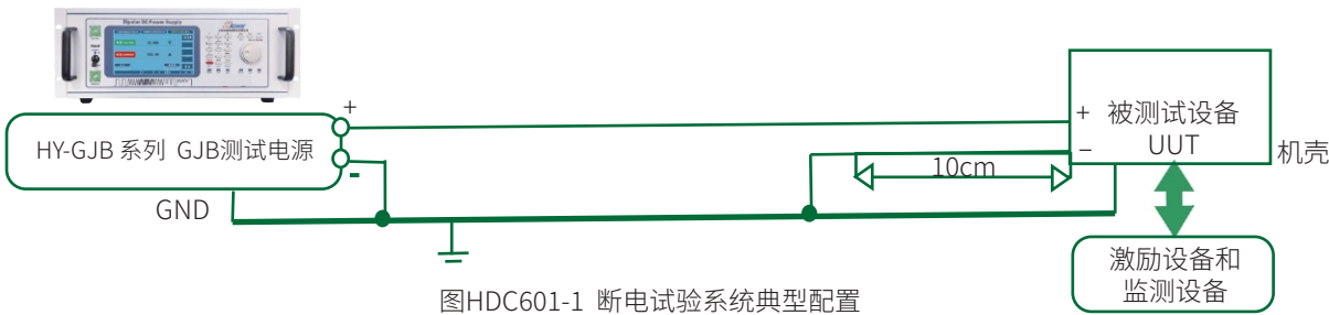
图HDC601-1 断电试验系统典型配置
