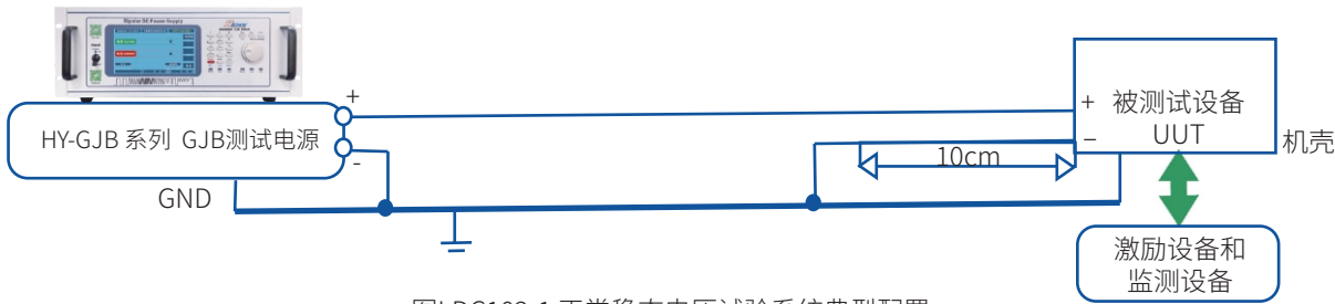
图LDC102-1 正常稳态电压试验系统典型配置
