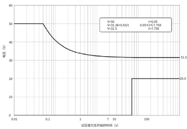
GJB 181B-2012 图14 28V直流非正常工作电压极限
