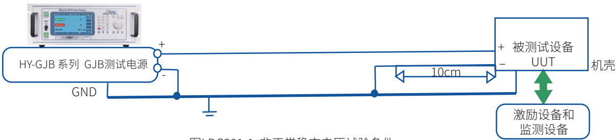
图LDC301-1 非正常稳态电压试验条件
