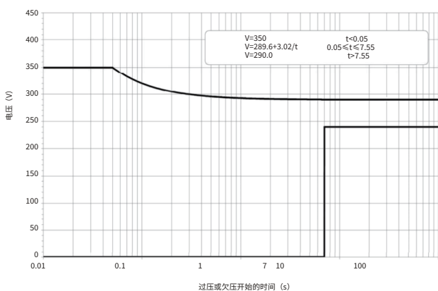
GJB 181B-2012 图17 270V直流非正常工作电压极限
