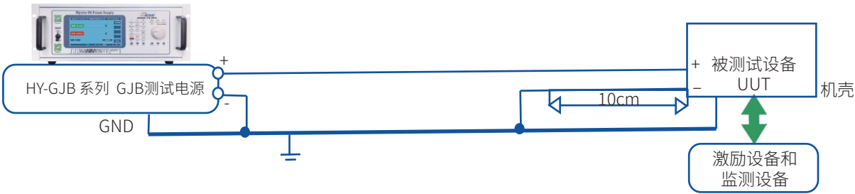
图LDC601-1 断电试验系统典型配置
