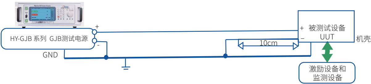
图LDC501-1 起动电压瞬变试验系统典型配置
