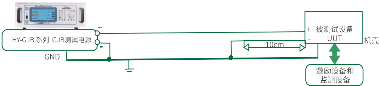
图HDC301-1 非正常稳态电压试验条件
