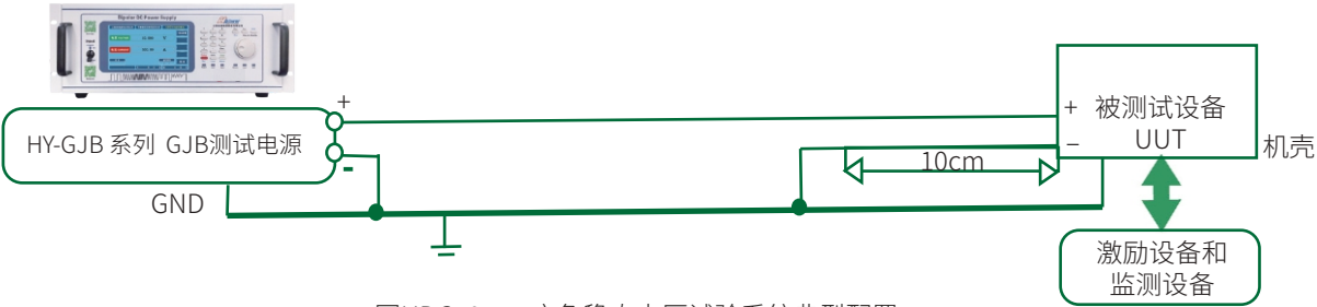
图HDC401-1 应急稳态电压试验系统典型配置
