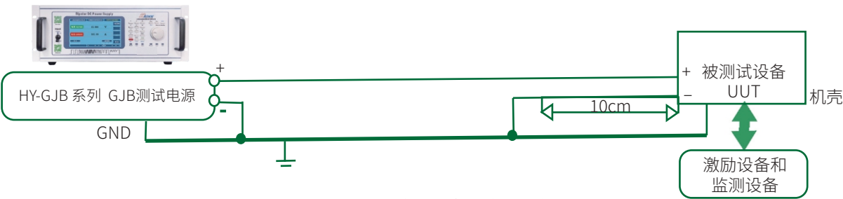
图HDC501-1 起动电压瞬变试验系统典型配置
