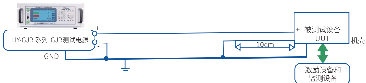
图LDC103-1 电压畸变频谱试验系统典型配置1
