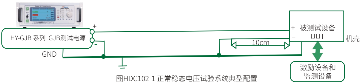
图HDC102-1 正常稳态电压试验系统典型配置
