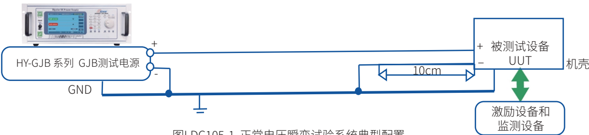
图LDC105-1 正常电压瞬变试验系统典型配置
