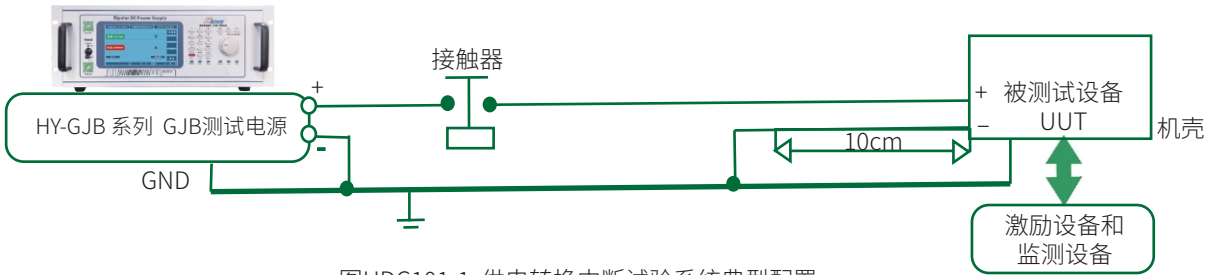
图HDC101-1 供电转换中断试验系统典型配置
