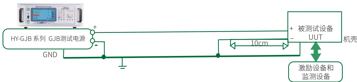
图HDC302-1 非正常电压瞬变试验系统典型配置
