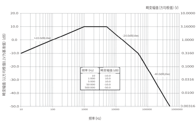
GJB 181B-2012 图16 270V直流电压最大畸变频谱
